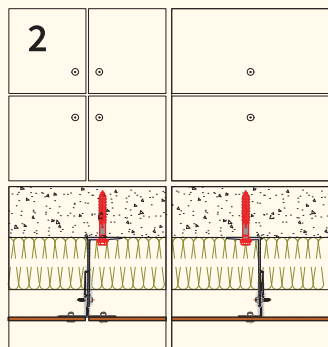
2. 'L-T Profile' system
